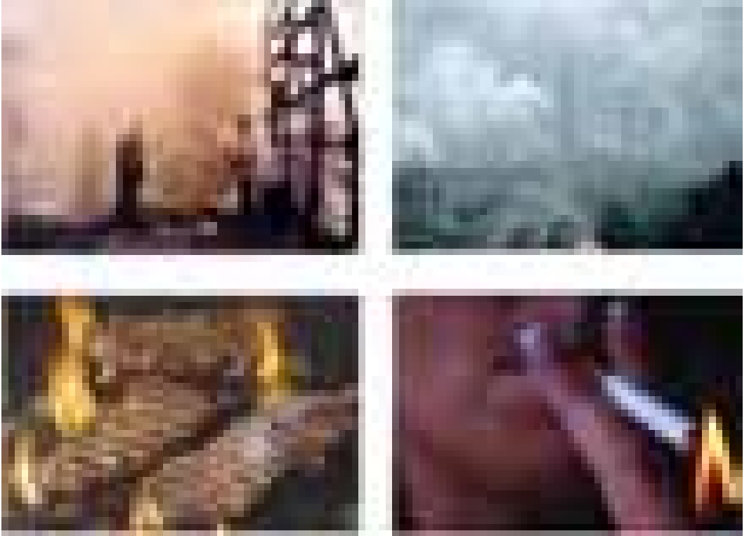
Figura 2 Principales hidrocarburos aromáticos policíclicos (HAP)
